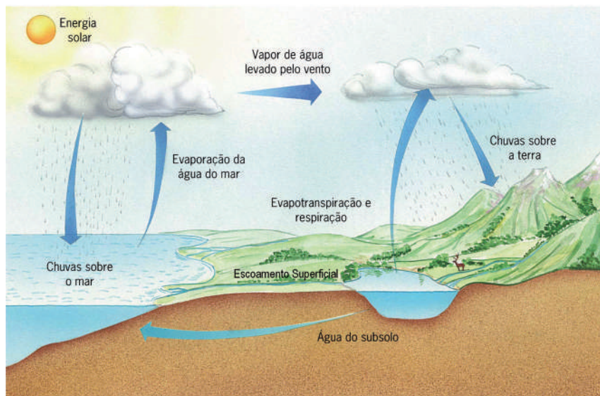
Figura 2 – Esquema ciclo da água
